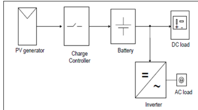
Şekil 2.1. Fotovoltaiik sistemlerin iç yapısının genel gösterimi
